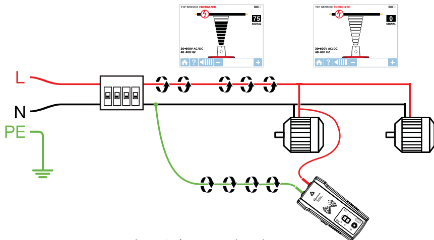
Figura 3.1b: Trasmittore impostato
