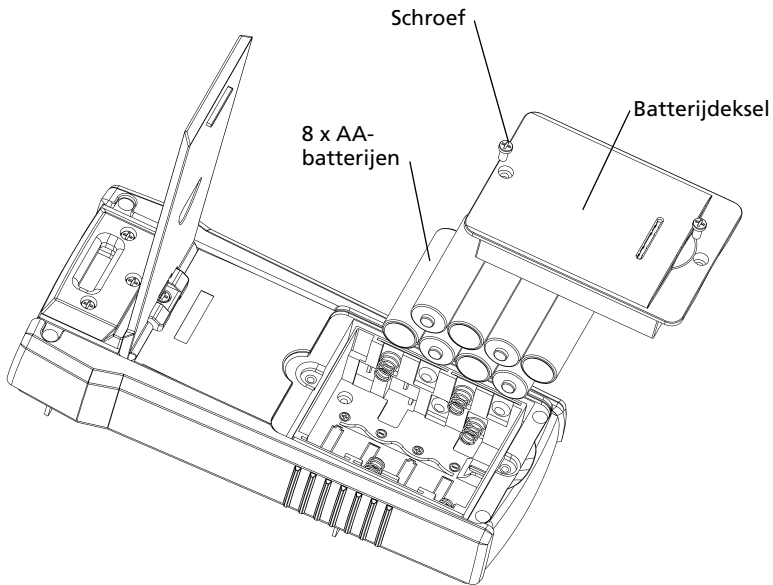
Afbeelding 5.1a: Zenderbatterijen vervangen
