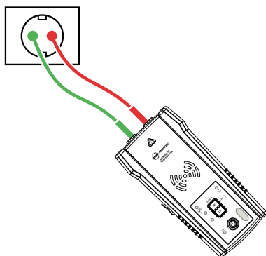
Figur 3.3a: Förenklad direktanslutning
