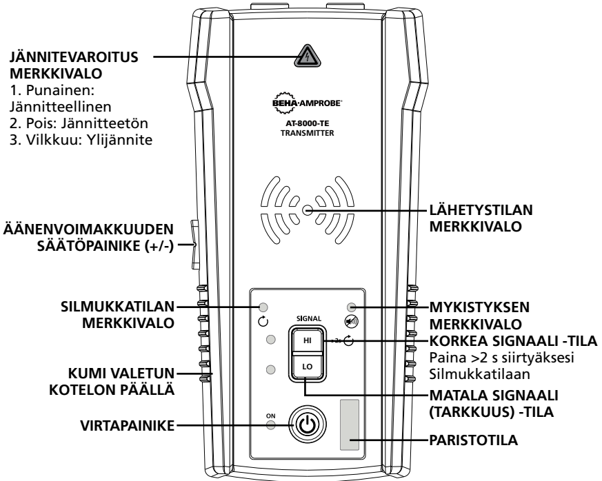
Kuva 2.3: AT-8000-TE-lähettimen yleiskatsaus
