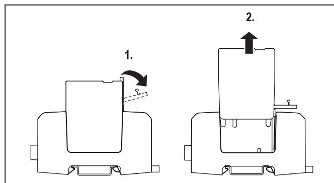
Bild 8.2 Überspannungsableiter entfernen
