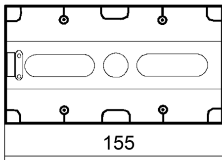
Mått ritning
