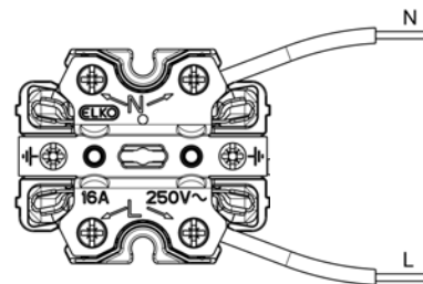
Kopplingsschema
