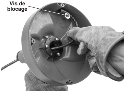
Figure 11 – Amarrage de l'extrémité du câble
