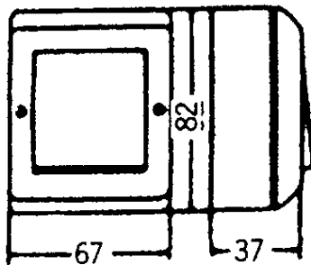
Måttritning
