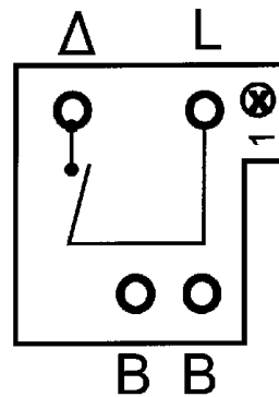
Kopplingsschema
