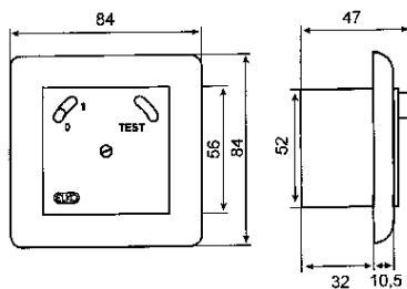
Måttritning
