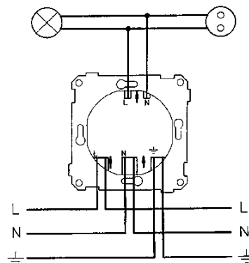
Kopplingsschema
