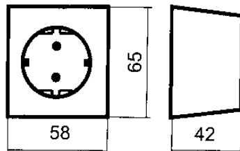
Måttritning
