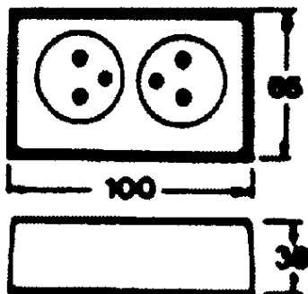
Måttritning
