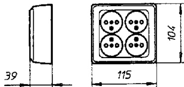
Måttritning
