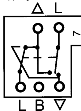
Kopplingschema
