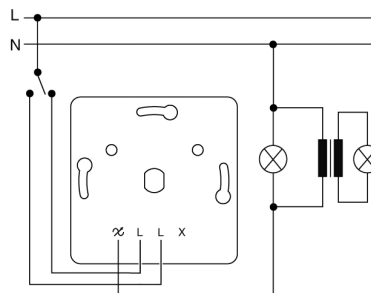
Kopplingsschema
