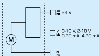
Ställdon serie ARA659
