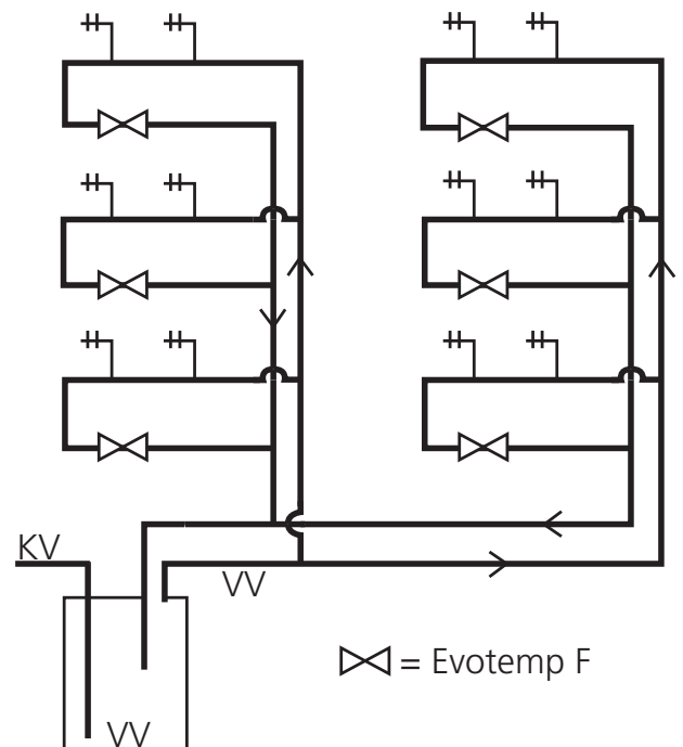
Kopplingschema/Wiring diagramAsennusesimerkki
