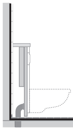
Tätskikt bakom WC-modul i våtrum.
