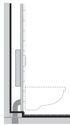
Tätskikt bakom WC-modul i WC-rum.
